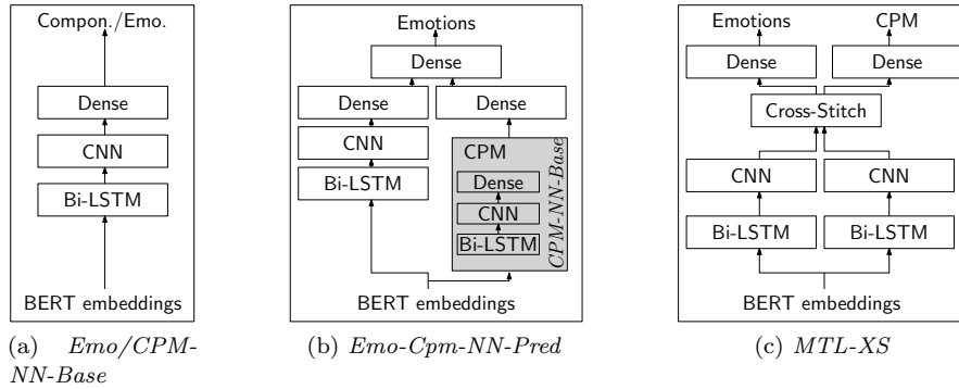
Abbildung 2: Neuronale Modellarchitekturen zur Vorhersage von Emotionskomponenten und Emotionen
