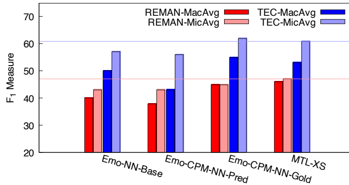
Abbildung 3: Ergebnisse der Emotionsklassifikation unter Berücksichtigung der Emotionskomponenten
