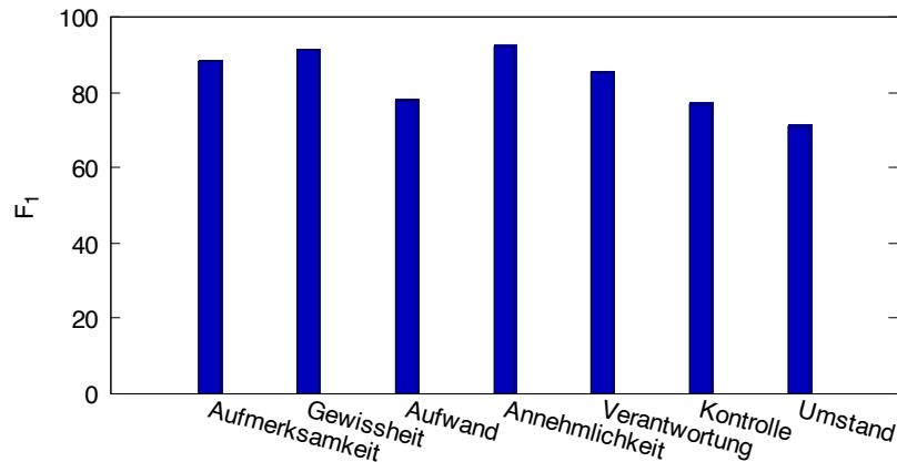
Abbildung 5: Ergebnisse der Vorhersage der Appraisaldimensionen mit Hilfe einer 3 \times 10 -fach Kreuzvalidierung
